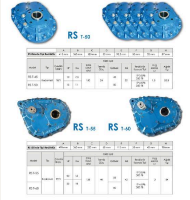
RS KADEMELİ REDÜKTÖR
