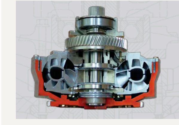
Tork Konvertör
